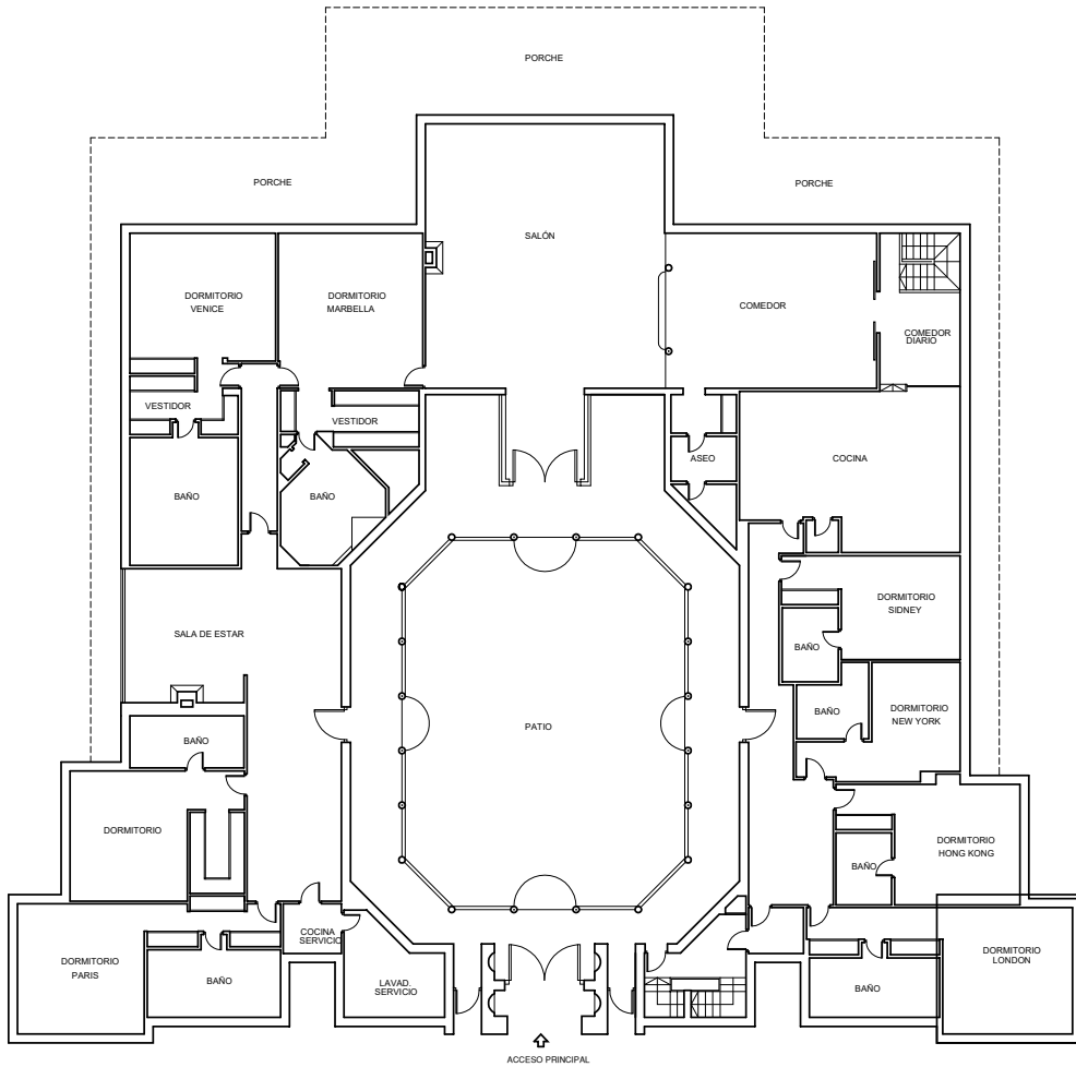
PLANTA BAJA ACCESO 0 1 2 3 4 5 m
