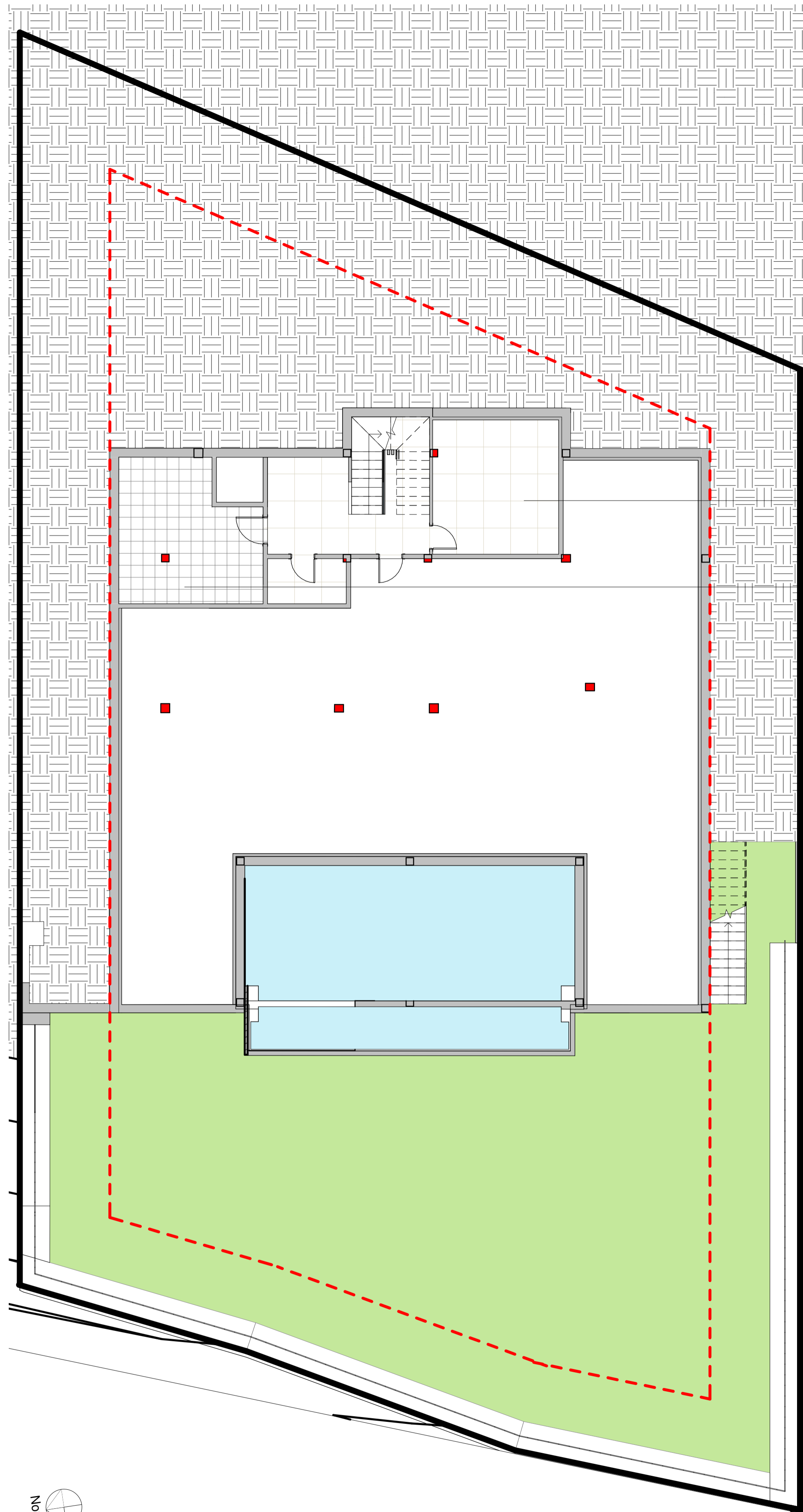
1 VC05 - Solados Planta sótano 1 : 100
