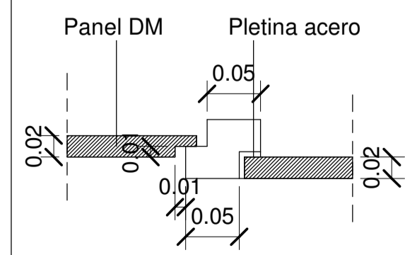
DETALLE FALSO TECHO REGISTRABLE
